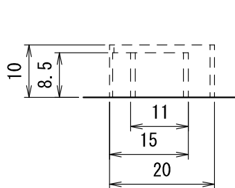
側面ロックアウト A 詳細 (1/1)
