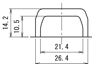
側面ロックアウト B 詳細 (1/1)
